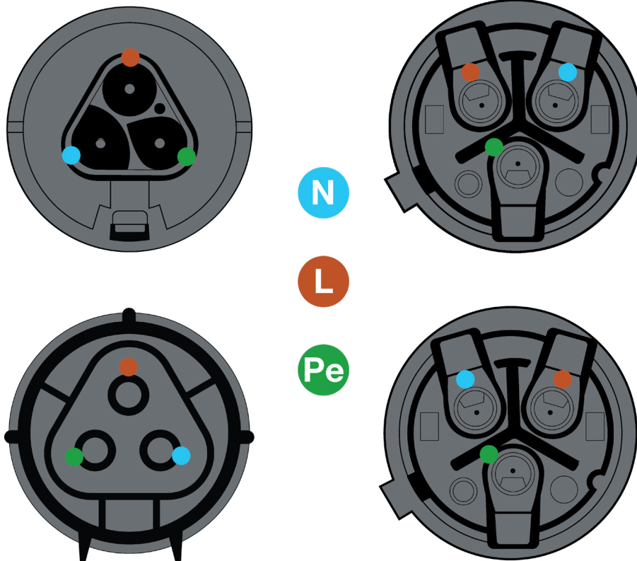
AC Power Plug (AC Stromanschluss)
